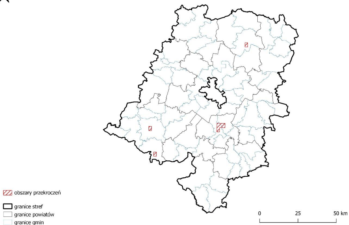
Rysunek 7.47. Zasięg obszarów przekroczeń poziomu docelowego B(a)P w pyłe zawieszonym PM10, określonego ze względu na ochronę zdrowia ludzi w województwie opolskim w 2023 roku [źródło: GIOŚ]
