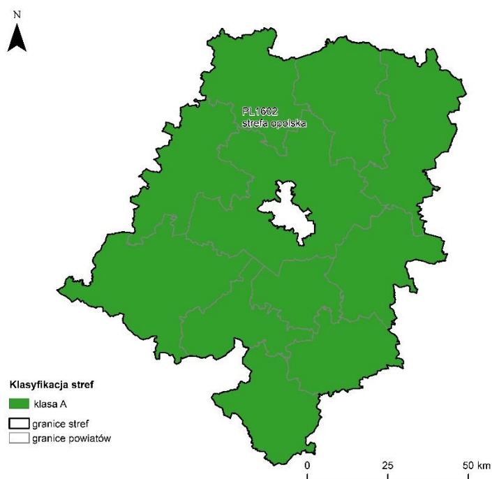
Rysunek 7.52. Klasyfikacja stref w województwie opolskim za 2023 rok dla NO x dla czasu uśredniania - rok, z uwzględnieniem kryteriów określonych w celu ochrony roślin [źródło: GIOŚ]
