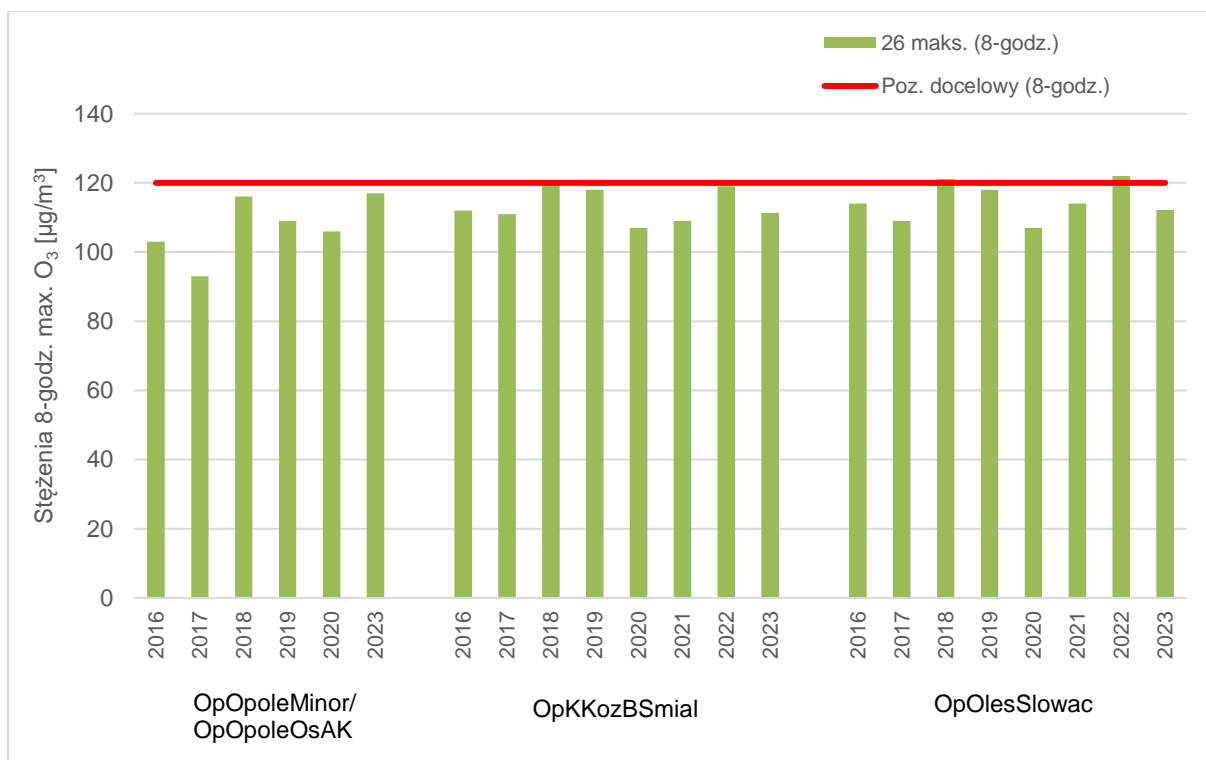
Rysunek 7.20. Przebieg 26-tych maksymalnych rocznych wartości dobowych maksimumów ze stężeń średnich 8-godzinnych O 3 , na poszczególnych stanowiskach pomiarowych w województwie opolskim, na tle poziomu docelowego w latach 2016 - 2023 [źródło: GIOŚ]
