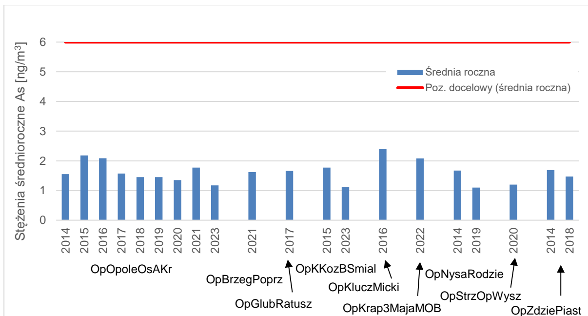
Rysunek 7.38. Przebieg wartości średnich rocznych stężeń As w pyłe zawieszonym PM10, na poszczególnych stanowiskach pomiarowych w województwie opolskim, na tle poziomu docelowego w latach 2014 - 2023 [źródło: GIOŚ]
