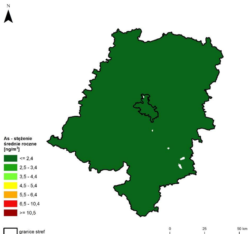
Rysunek 7.39. Rozkład przestrzenny wartości stężenia średniego rocznego As w pyłe zawieszonym PM10 w województwie opolskim w 2023 roku, opracowany z wykorzystaniem metody szacowania w oparciu o wyniki modelowania jakości powietrza dla roku 2023 wykonanego przez IOŚ-PIB [źródło: GIOŚ, IOŚ-PIB]
