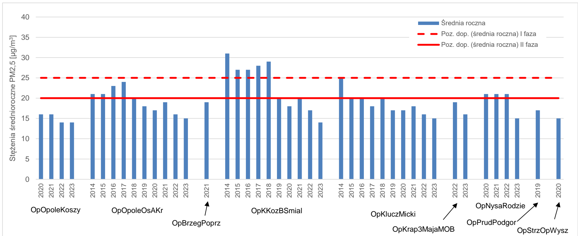
Rysunek 7.33. Przebieg wartości stężenia średniego rocznego pyłu zawieszonego PM 2,5 , na poszczególnych stanowiskach pomiarowych w województwie opolskim na tle poziomym dopuszczalnego w latach 2014 - 2023 [źródło: GIOŚ]
