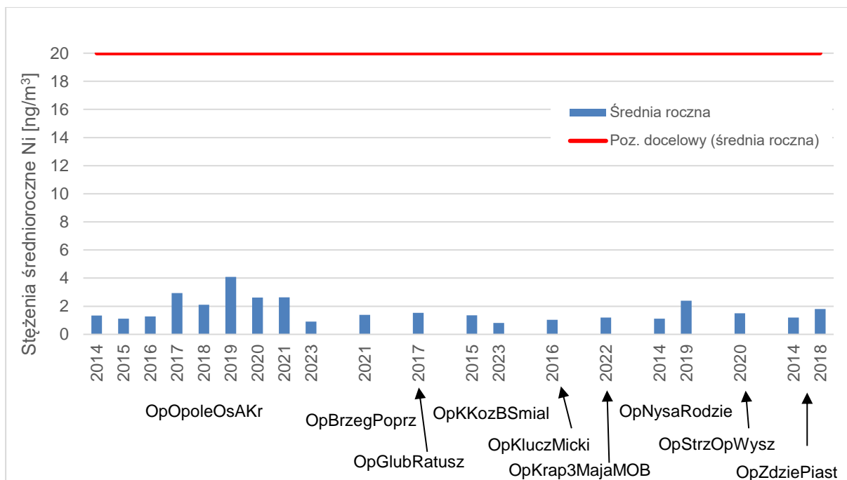
Rysunek 7.43. Przebieg wartości średnich rocznych stężeń Ni w pyłe zawieszonym PM10, na poszczególnych stanowiskach pomiarowych w województwie opolskim, na tle poziomu docelowego w latach 2014 - 2023 [źródło: GIOŚ]
