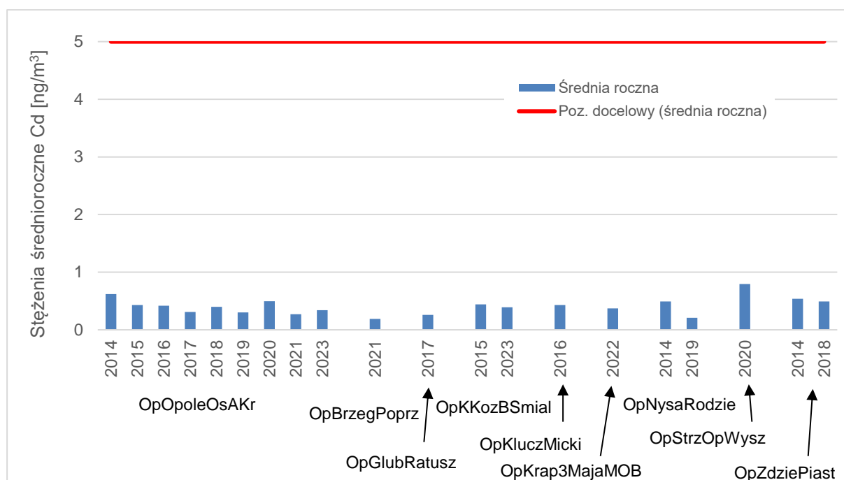
Rysunek 7.41. Przebieg wartości średnich rocznych stężeń Cd w pyłe zawieszonym PM10, na poszczególnych stanowiskach pomiarowych w województwie opolskim, na tle poziomu docelowego w latach 2014 - 2023 [źródło: GIOŚ]
