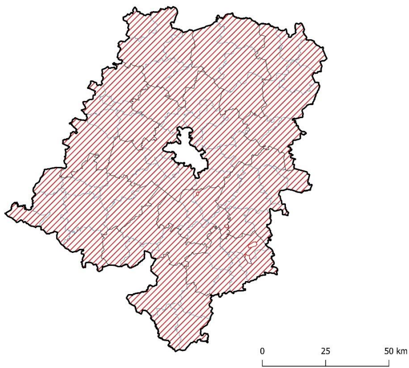
Rysunek 7.58. Zasięg obszarów przekroczeń poziomu celu długoterminowego (wskaźnika AOT40) dla O 3 ustanowionego ze względu na ochronę roślin w województwie opolskim w 2023 roku [źródło: GIOŚ]
