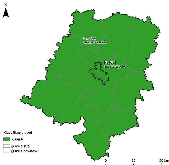
Rysunek 7.13. Klasyfikacja stref w województwie opolskim za 2023 rok dla tlenku węgla dla czasu uśredniania - 8 godz., z uwzględnieniem kryteriów określonych w celu ochrony zdrowia ludzi [źródło: GIOŚ]
