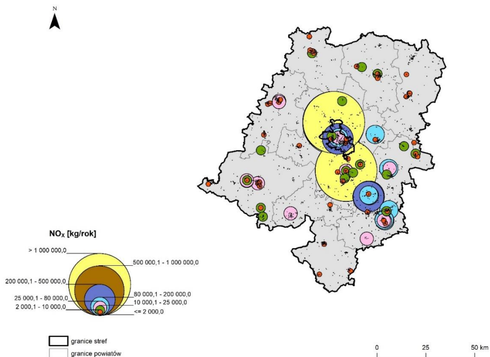
Rysunek 6.3. Lokalizacja punktowych źródeł emisji NO x na obszarze województwa opolskiego [opracowanie GIOŚ, źródło: KOBIZE / IOŚ-PIB]
