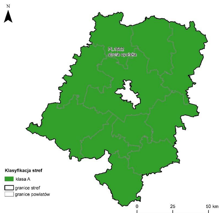
Rysunek 7.49 Klasyfikacja stref w województwie opolskim za 2023 rok dla SO 2 dla czasu uśredniania – pora zimowa, z uwzględnieniem kryteriów określonych w celu ochrony roślin [źródło: GIOŚ]
