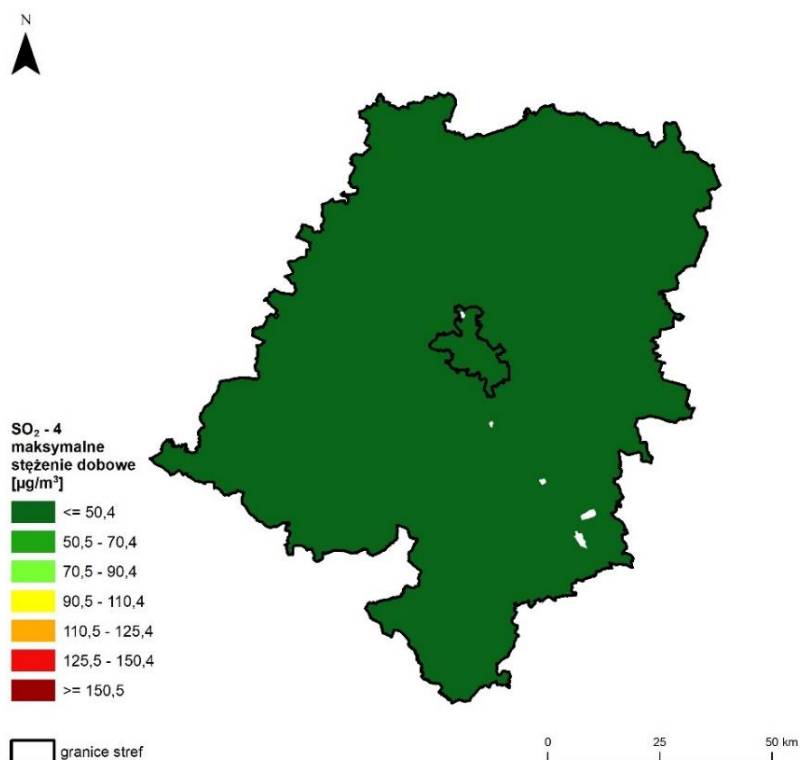
Rysunek 7.6. Rozkład przestrzenny 4 maksymalnej wartości stężenia 24-godzinne SO 2 w województwie opolskim w 2023 roku, opracowany z wykorzystaniem metody szacowania w oparciu o wyniki modelowania jakości powietrza dla roku 2023 wykonanego przez IOŚ-PIB [źródło: GIOŚ, IOŚ-PIB]
