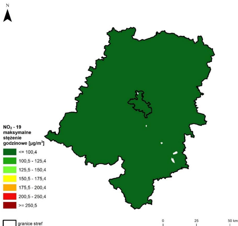
Rysunek 7.11. Rozkład przestrzenny 19 maksymalnej wartości stężenia 1-godzinowego NO 2 w województwie opolskim w 2023 roku, opracowany z wykorzystaniem metody szacowania w oparciu o wyniki modelowania jakości powietrza dla roku 2023 wykonanego przez IOŚ-PIB [źródło: GIOŚ, IOŚ-PIB]
