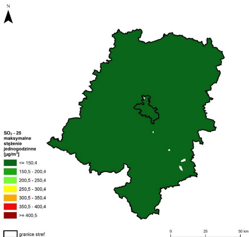
Rysunek 7.5. Rozkład przestrzenny 25 maksymalnej wartości stężenia 1-godzinne SO 2 w województwie opolskim w 2023 roku, opracowany z wykorzystaniem metody szacowania w oparciu o wyniki modelowania jakości powietrza dla roku 2023 wykonanego przez IOŚ-PIB [źródło: GIOŚ, IOŚ-PIB]
