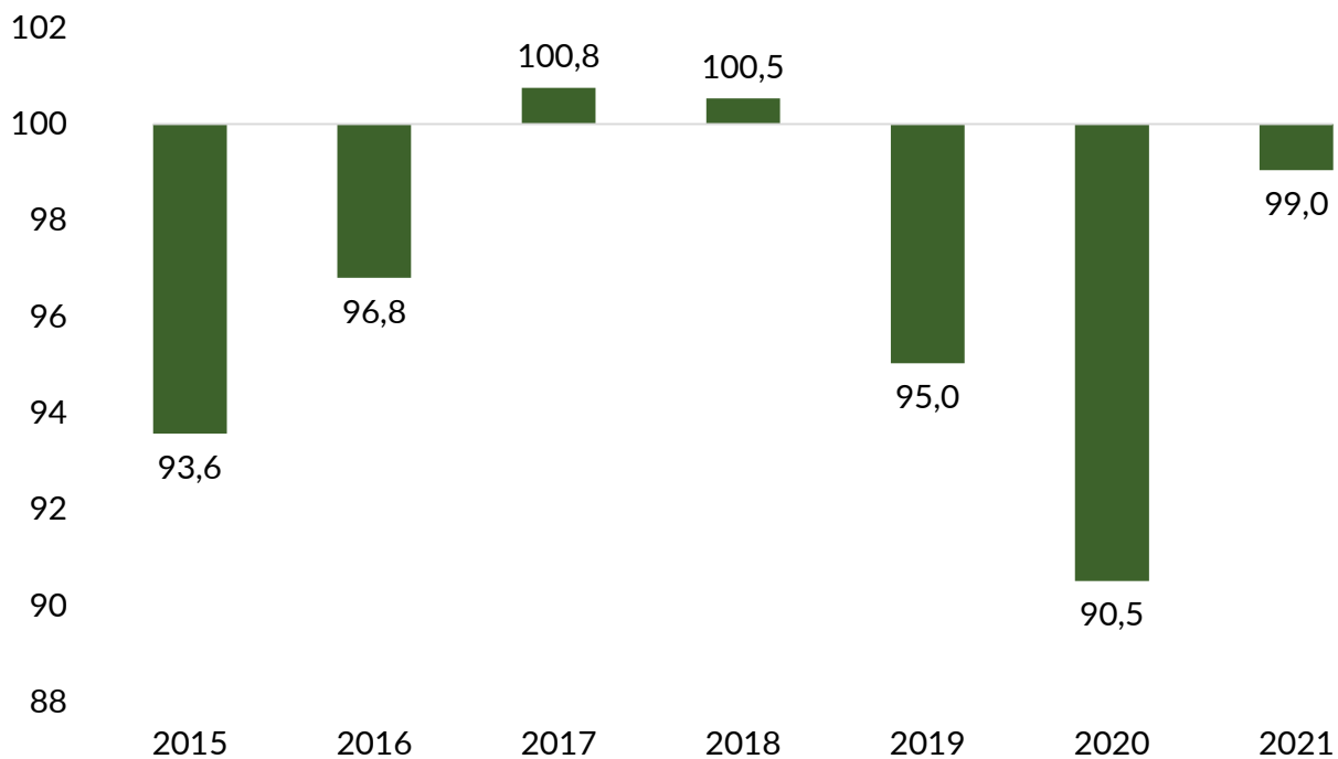
Dynamika emisji CO 2 (2010=100)
