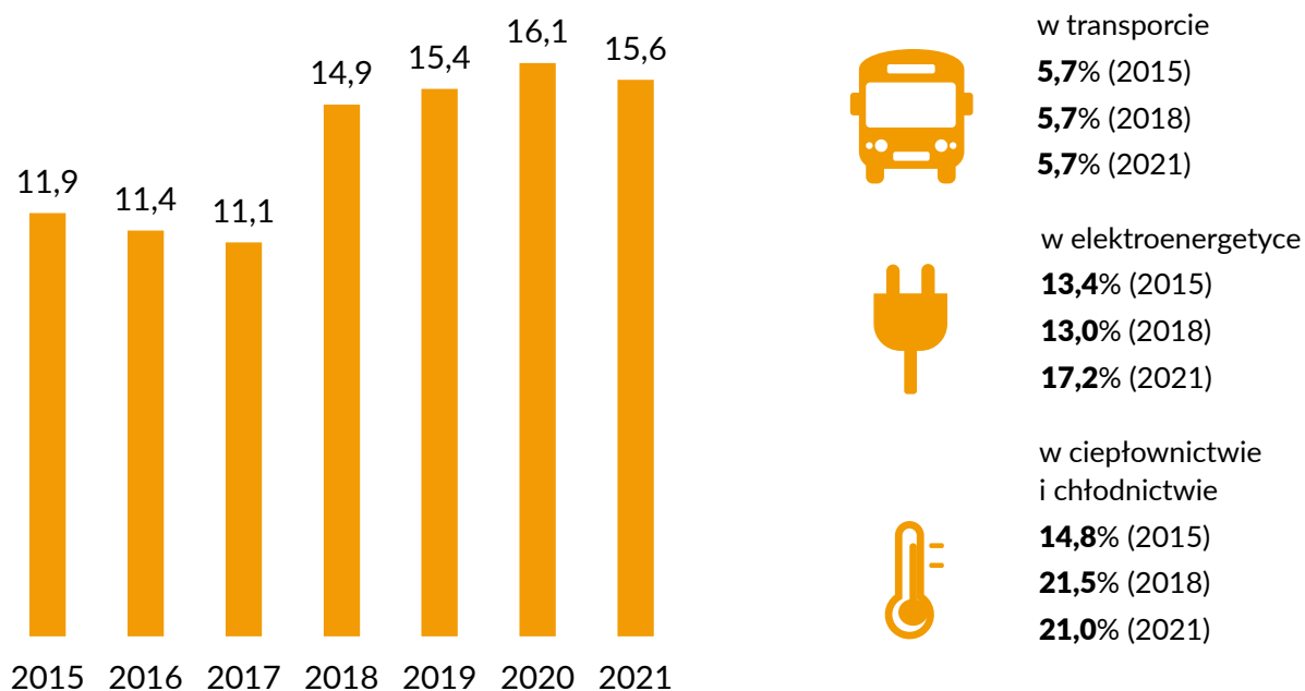
Udział energii ze źródeł odnawialnych w końcowym zużyciu energii brutto (%)
